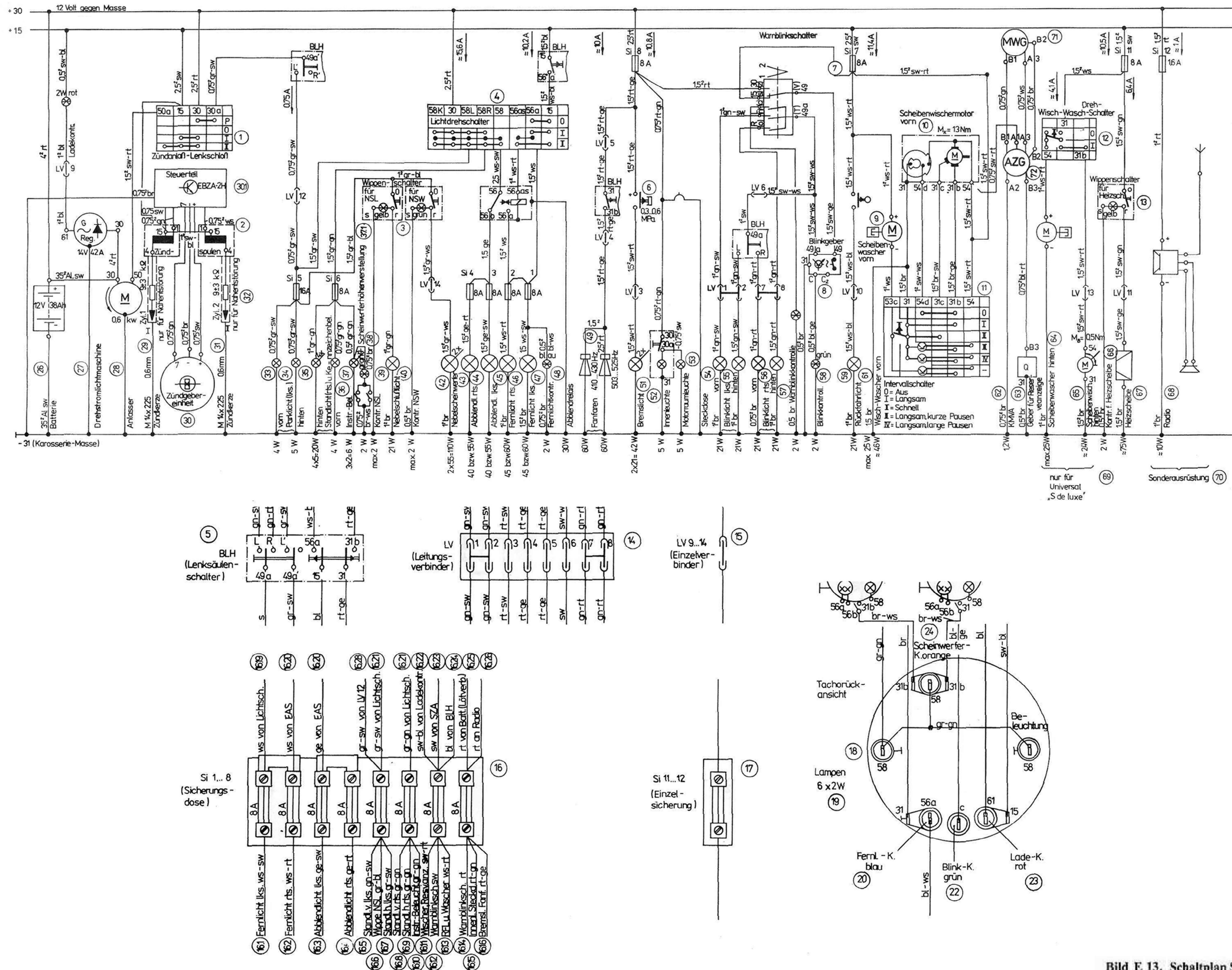
Bild E 13. Schaltplan S de luxe, Sonderwunsch
