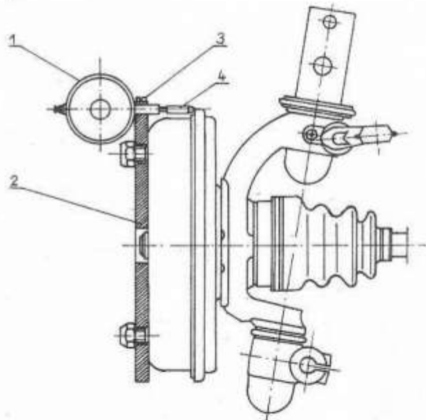
Bild F 9. Meßmethode zur Prüfung des Radlagerspieles
