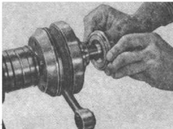
Bild M 2. Aufschieben der Kolbenringabdichtung
