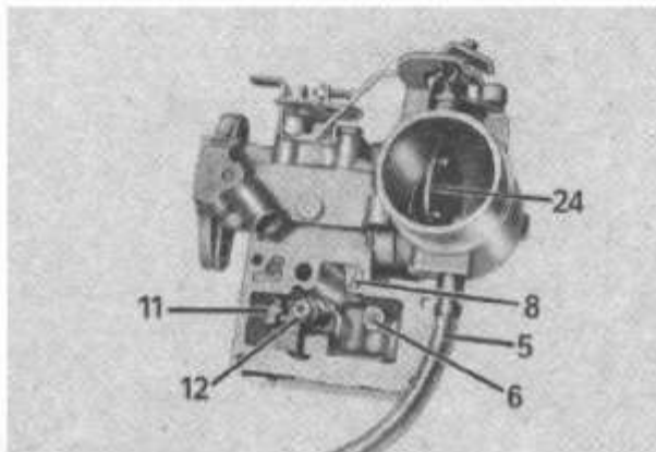
Bild M 4. Vergaser mit Anreicherungs-system
