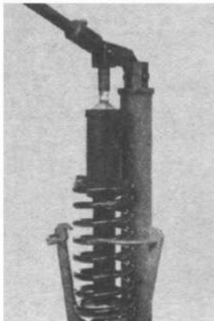
Bild F 12. Federbein in Montagevorrichtung eingelegt
