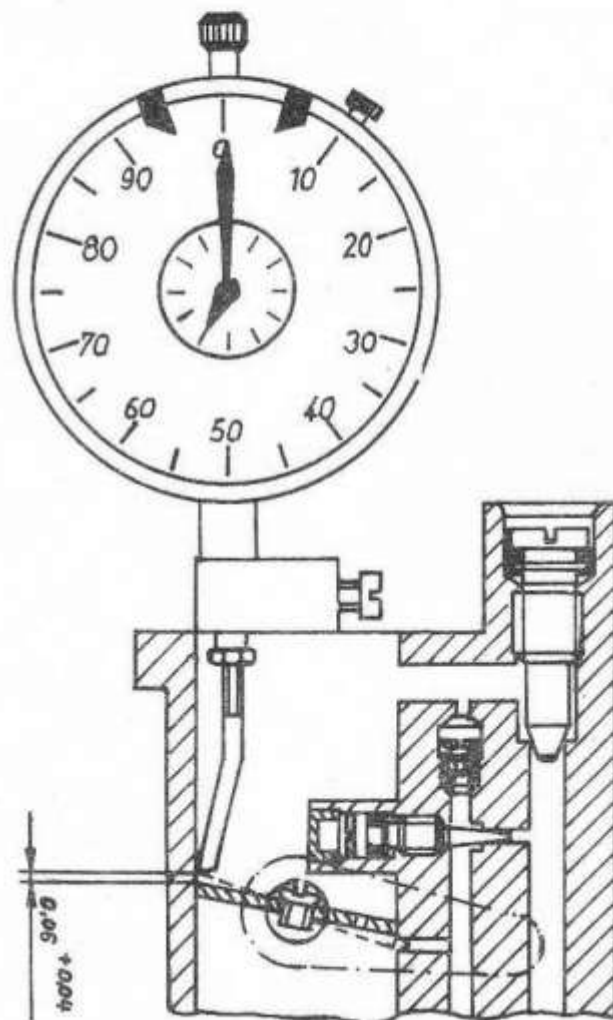
Bild M 9. Einstellung der Drosselklappe
