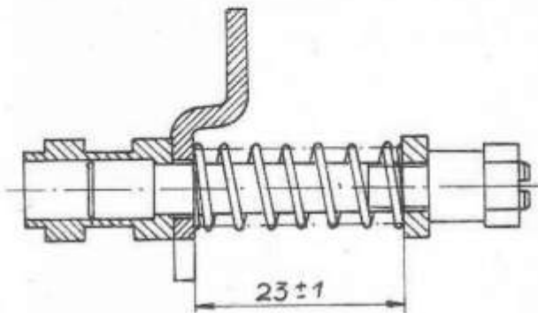
Bild M 11. Justiermaß des Stößels
