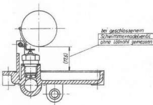
Bild M 7. Schwimmereinstellmaß
