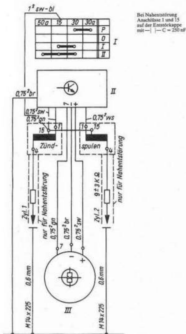
Bild E 8. Ergänzungsschaltplan für elektronische Batteriezündanlage (EBZA-2H)
