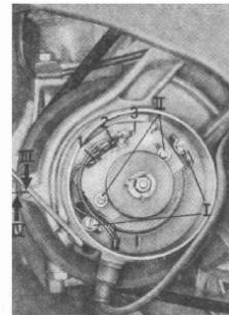
Bild E4. Gebergehäuse mit Gebereinheit
