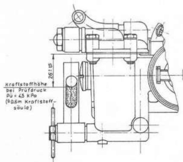
Bild M 8. Kraftstoffhöhe im Schwimmergehäuse
