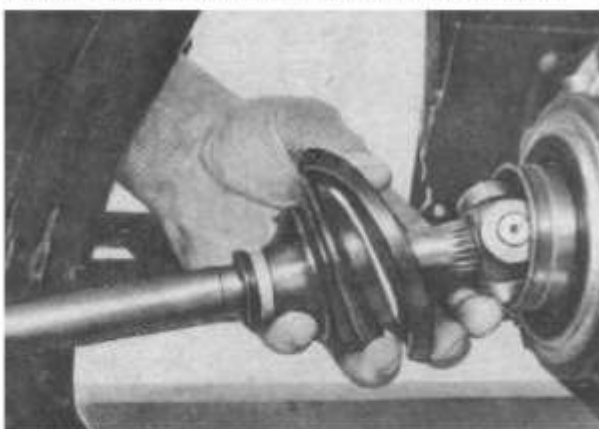
Bild F 4. Tripodegelenk in das Vorderachswellenrad schieben
