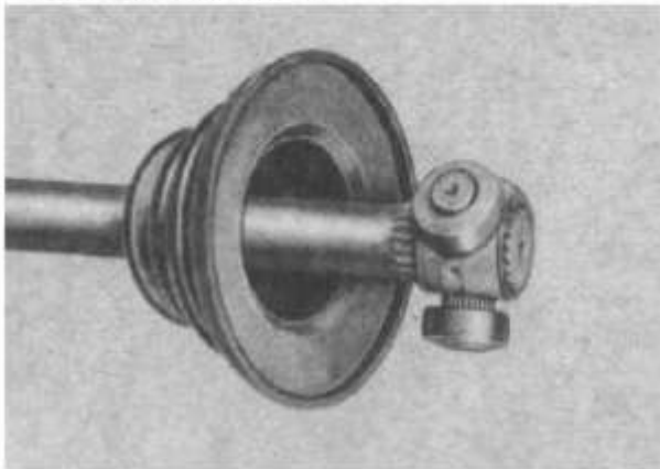
Bild F 7. Zapfenstern mit Nadelrollen
