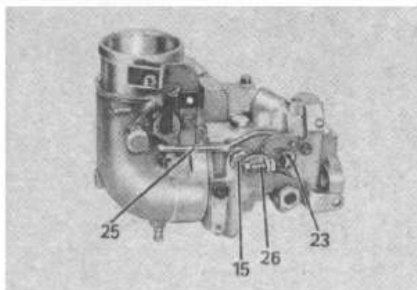
Bild M 5. Vergaser (linke Seite)
