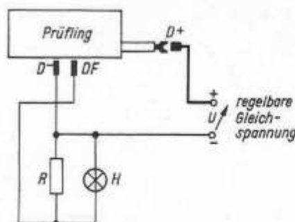
Bild E 11. Prüfschaltung am elektronischen Spannungsregler
