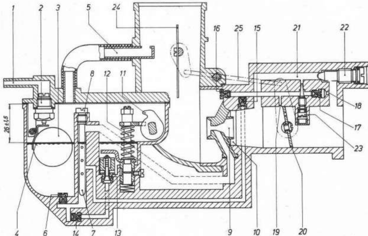
Bild M 3. Schematischer Längsschnitt des Vergasers 28 H1-1
