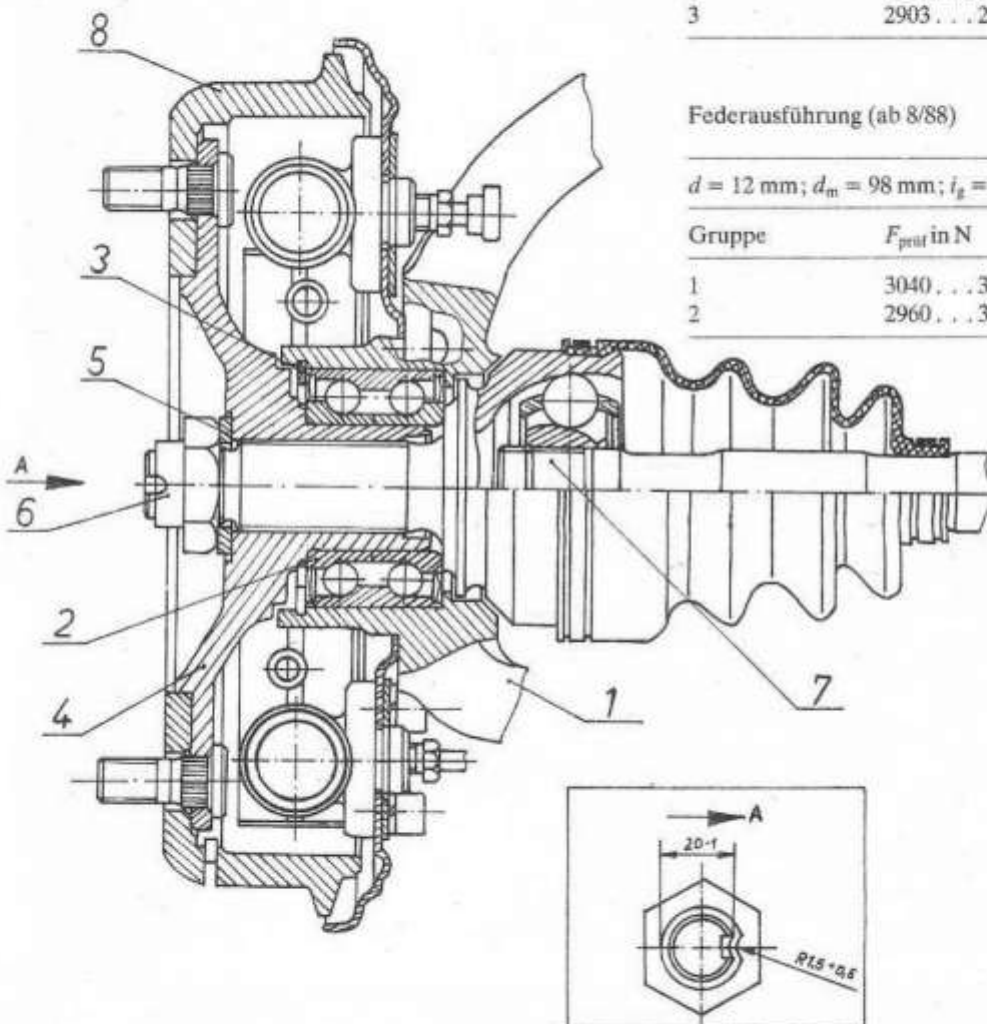
Bild F1. Radantrieb, vollst.
