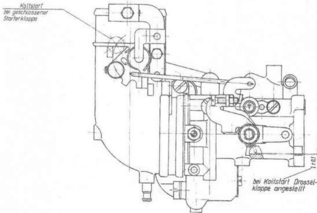
Bild M 10. Einstellung der Drosselklappe bei Kaltstart
