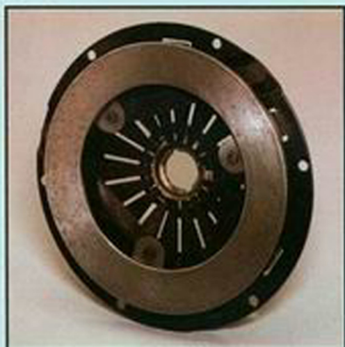
Kupplung T 160 mit Bandmitnahme und Kupplungsscheibe 160 DBR mit Drehschwingungsdämpfer – Dadurch weiches Einkuppeln beim Anfahren und Gangwechsel – Verringerung des Verschleißes des Nabenprofils –
